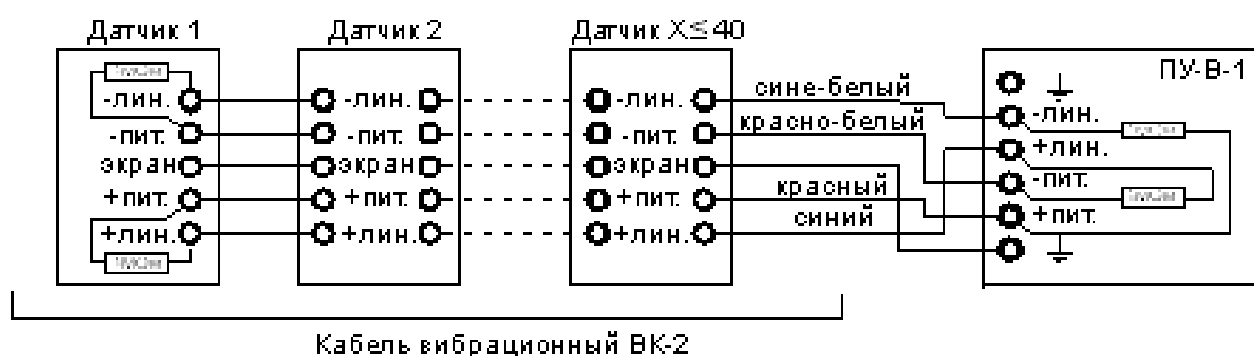
Рисунок 1 - Подключение кабеля к ПУ-В-1
